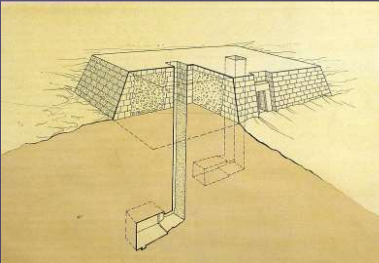
Schema di una Mastaba
